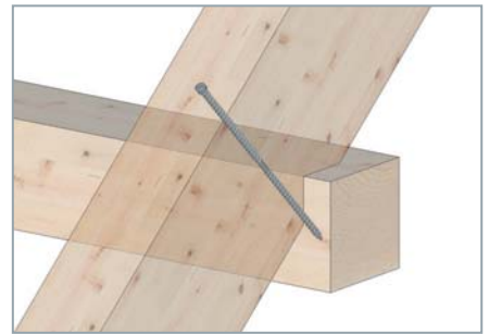
Sparren-Pfettenverbindung
