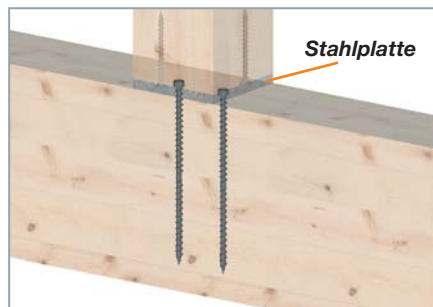
Ableitung starker Druckkräfte
