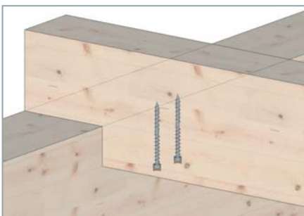
Verstärkung von Querschnittschwächungen
