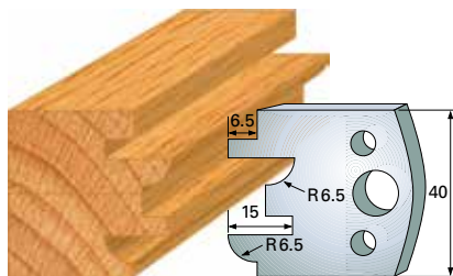
Konterprofil / Counter profile
