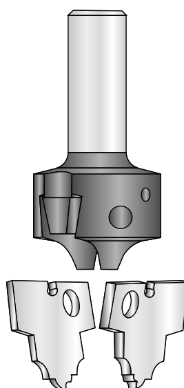
Grundkörper B Tool body B
